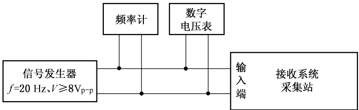
图 3 接收系统试验线路
