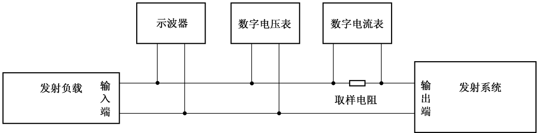
图 2 发射系统试验线路
