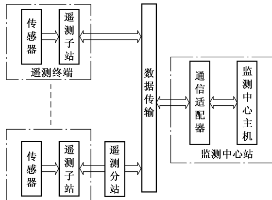
图 1 有线遥测总线结构、主从工作方式图
