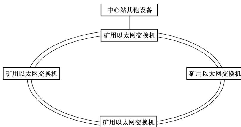
图 2 有源光网络双环结构
