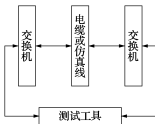
图 7 基于有源网络的矿用以太网电缆最大传输距离测试
