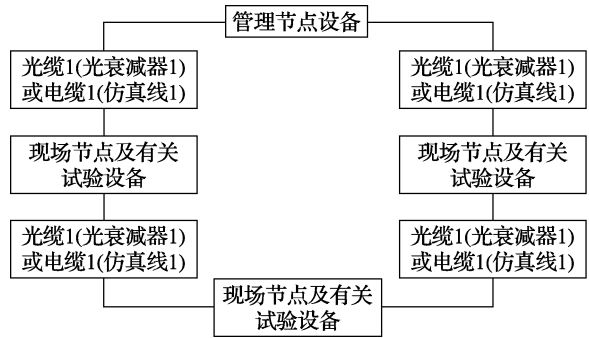
图 11 环形系统设备连接
