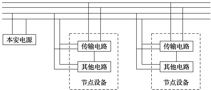
图 7 统一供电法
