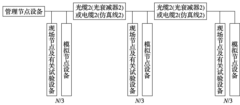
图 10 总线形系统设备连接
