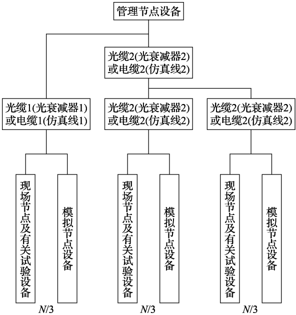
图 9 树形系统设备连接
