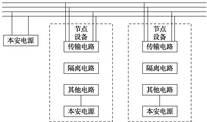
图 8 隔离供电法
