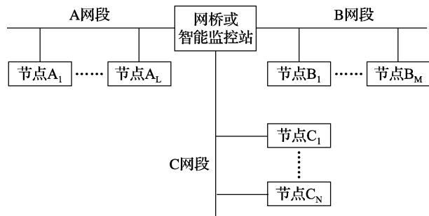
图 5 分段法
