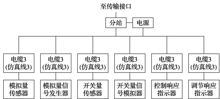
图 4 分站设备连接
