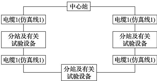
图 2 环形系统设备连接
