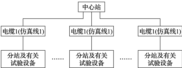
图 3 星形系统设备连接
