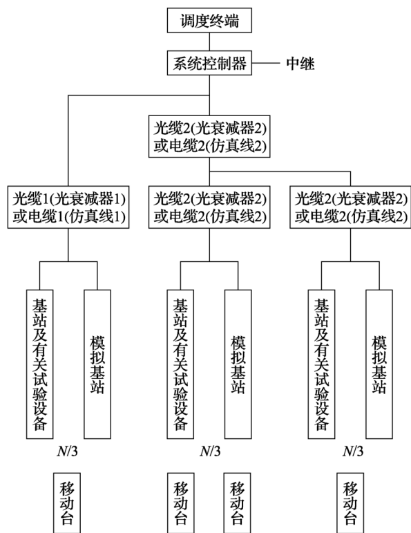
图 1 树形系统设备连接
