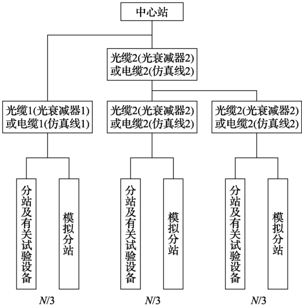
图 1 树形系统设备连接
