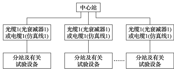
图 3 星形系统设备连接
