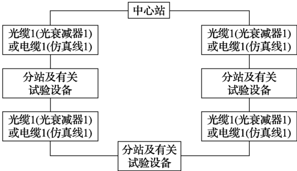
图 2 环形系统设备连接
