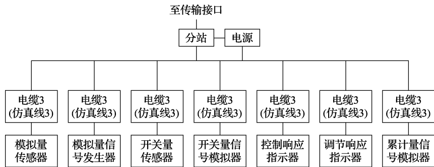
图 4 分站设备连接
