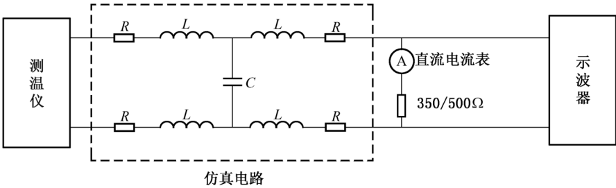
图 1 传输距离测试示意图
