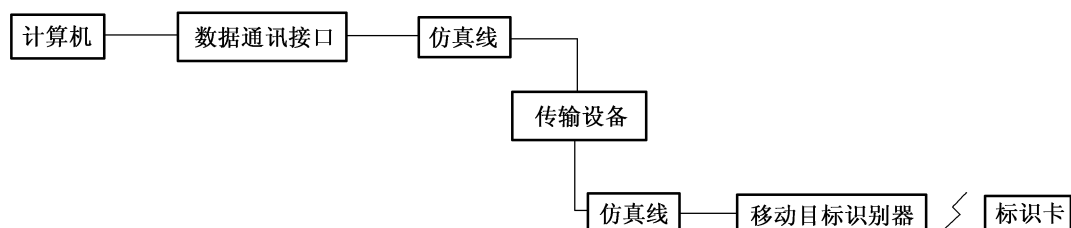
图 2 试验连接方式二
