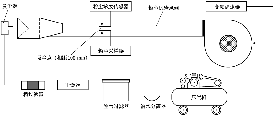
图 1 粉尘试验风洞试验系统
