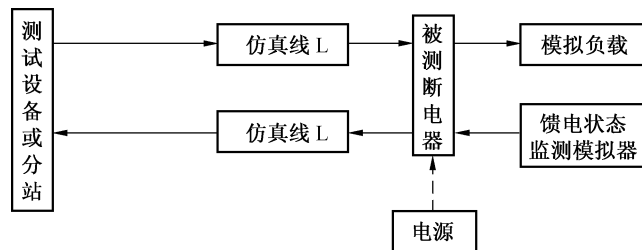
图 1 试验线路
