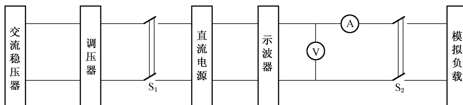
图 1 试验线路
