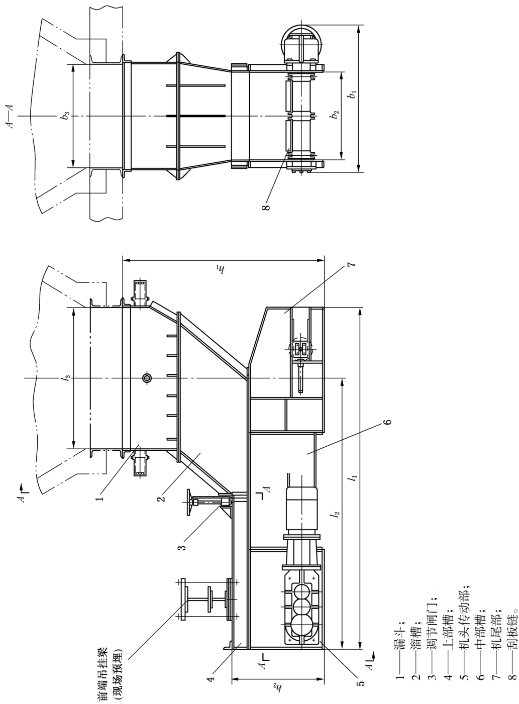
图1 链式刮板给料机结构尺寸简图
