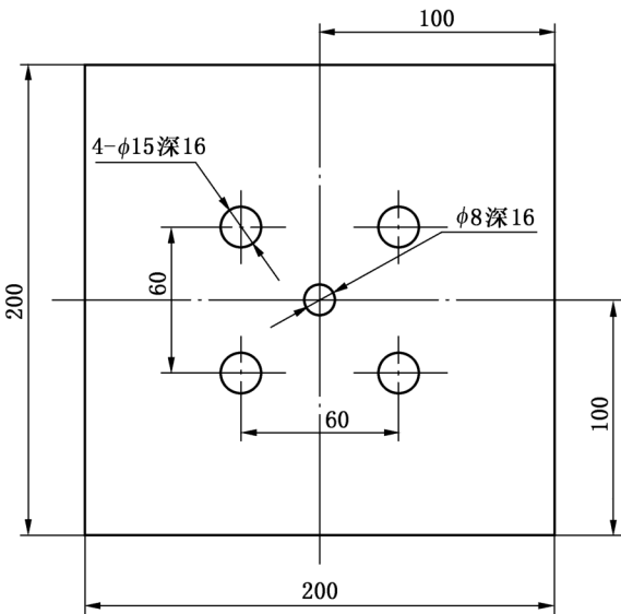
图 1 铁板平面图
