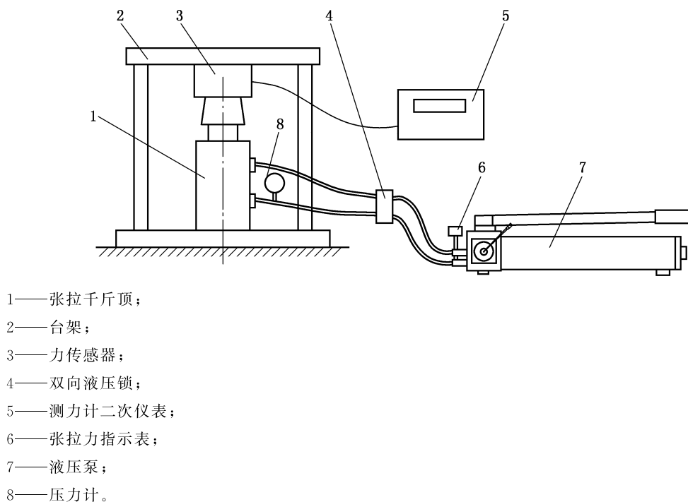
图 1 测试装置
