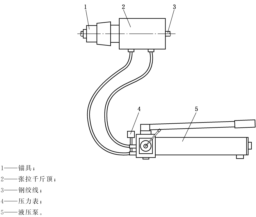
图 2 退锚试验
