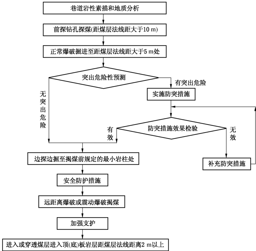
图 1 石门揭煤工艺流程
