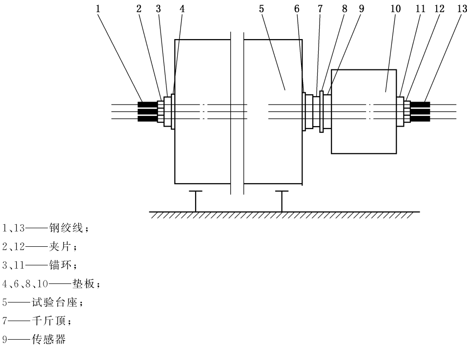
图 1 静载试验组装形式
