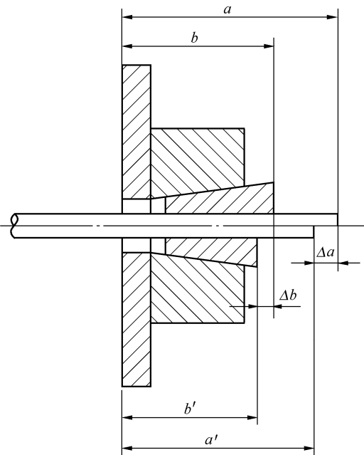
图 2 内缩量计算图
