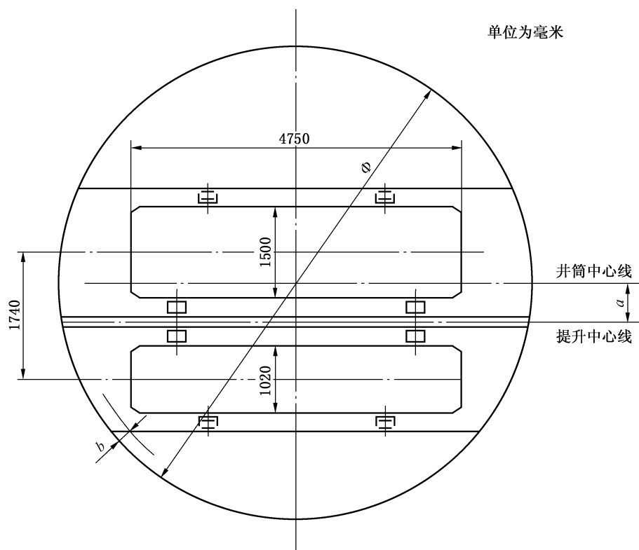
图 C.5 1t 矿车一层二车钢轨罐道罐笼
