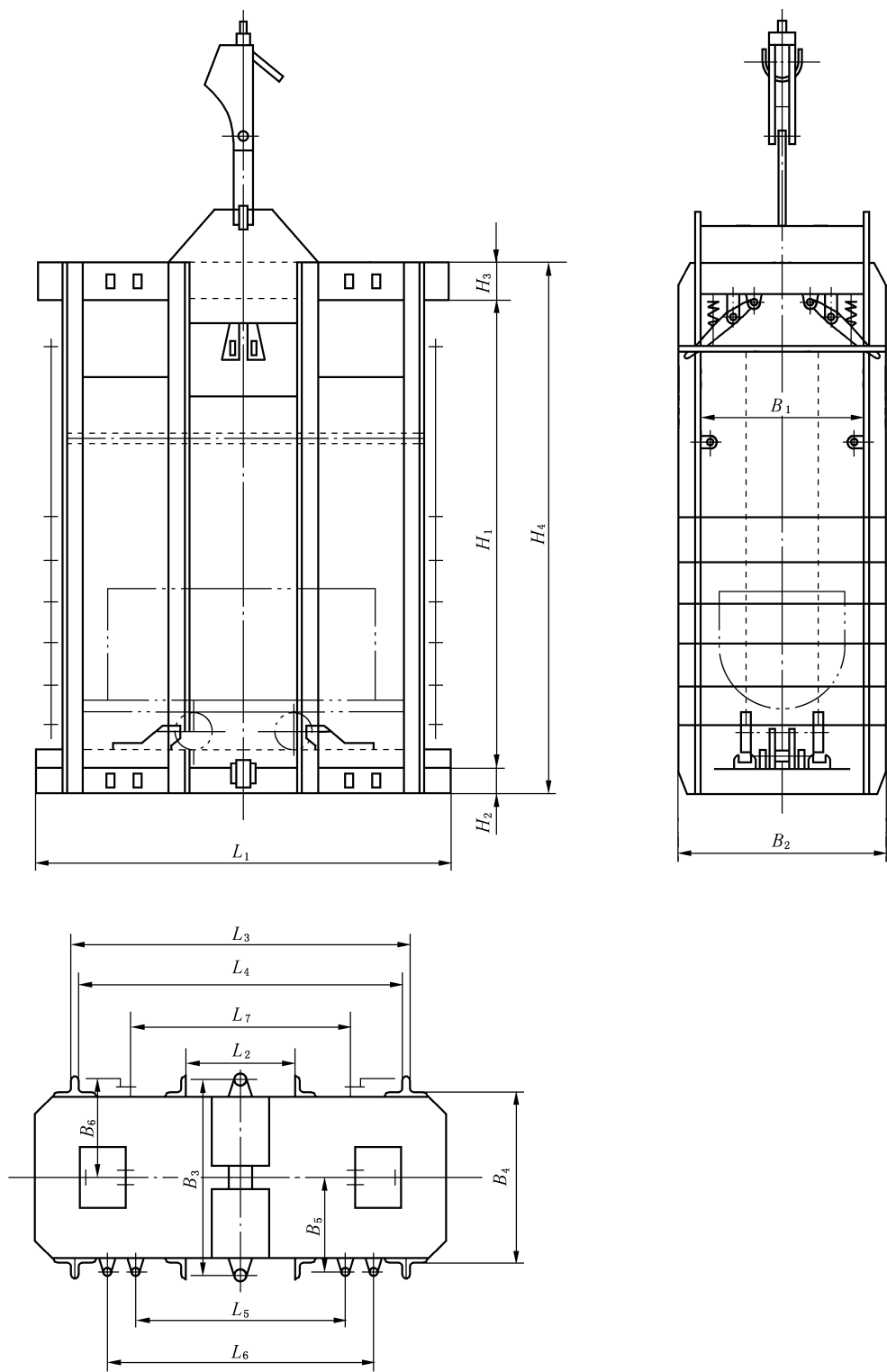
图 4 1t 矿车一层一车钢丝绳罐道罐笼
