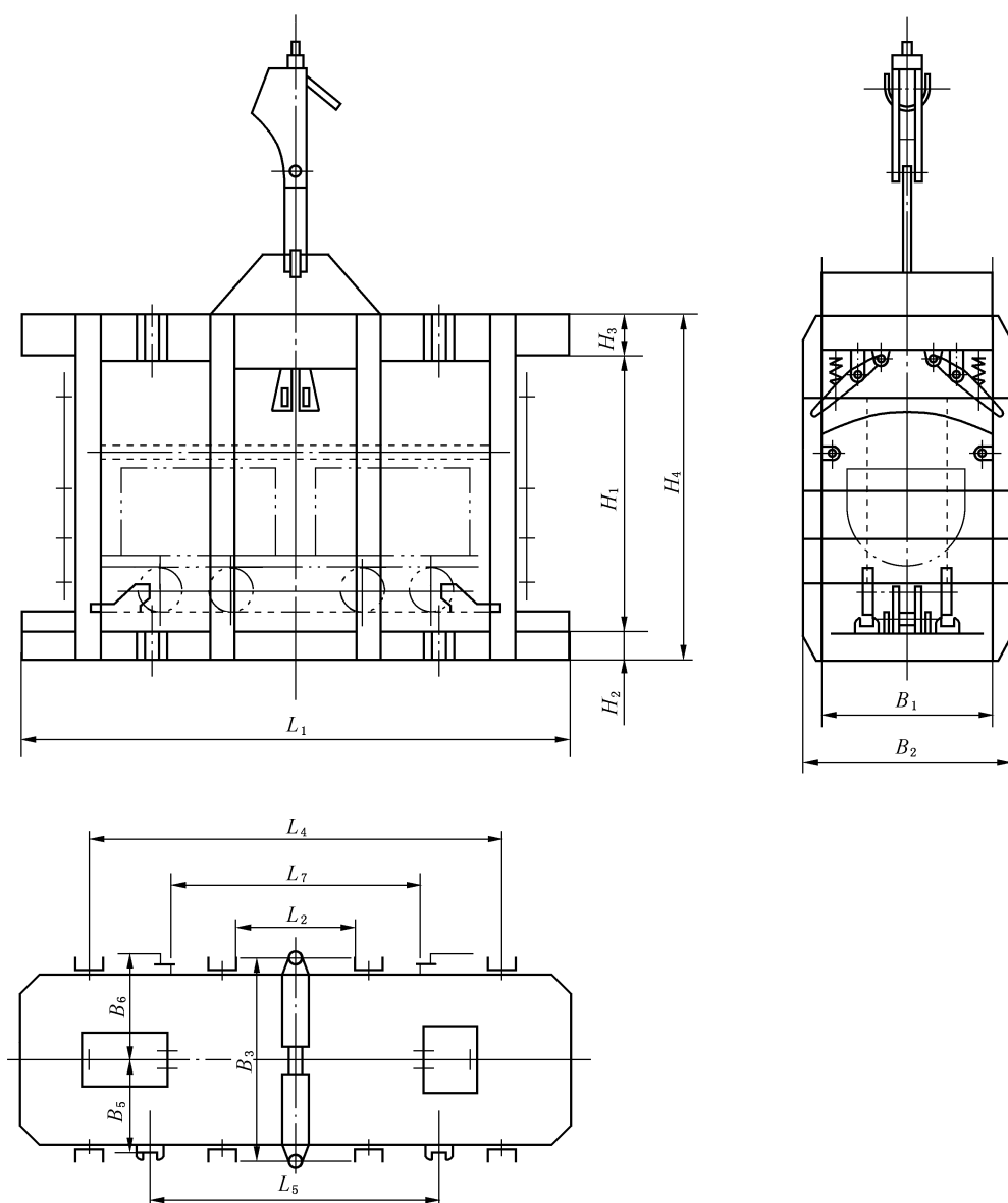
图 5 1t 矿车一层二车钢轨罐道罐笼
