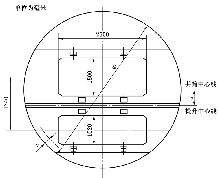
图 C.6 1t 矿车二层二车钢轨罐道罐笼
