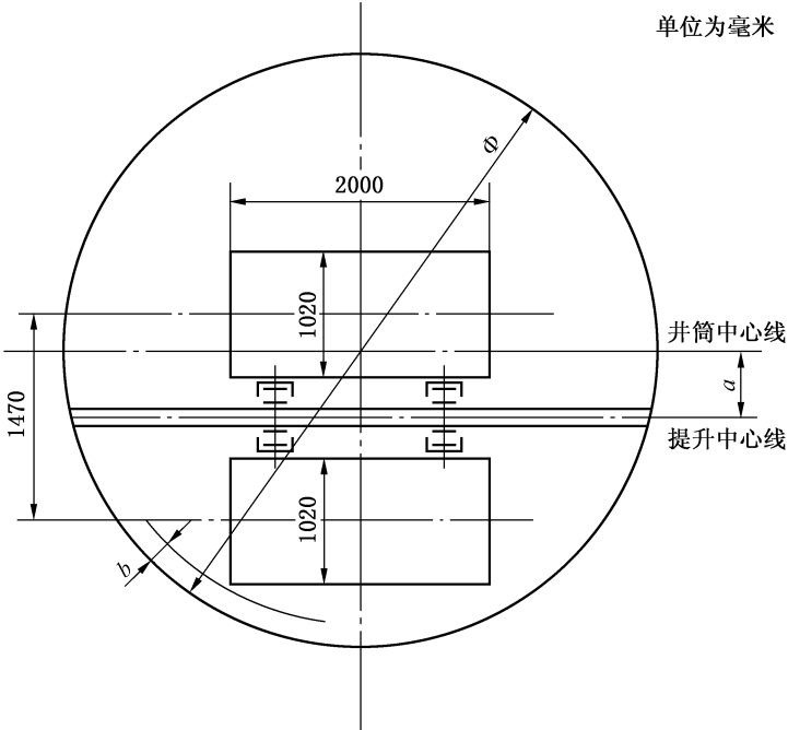
图 C.1 0.5t 矿车一层一车钢轨罐道罐笼
