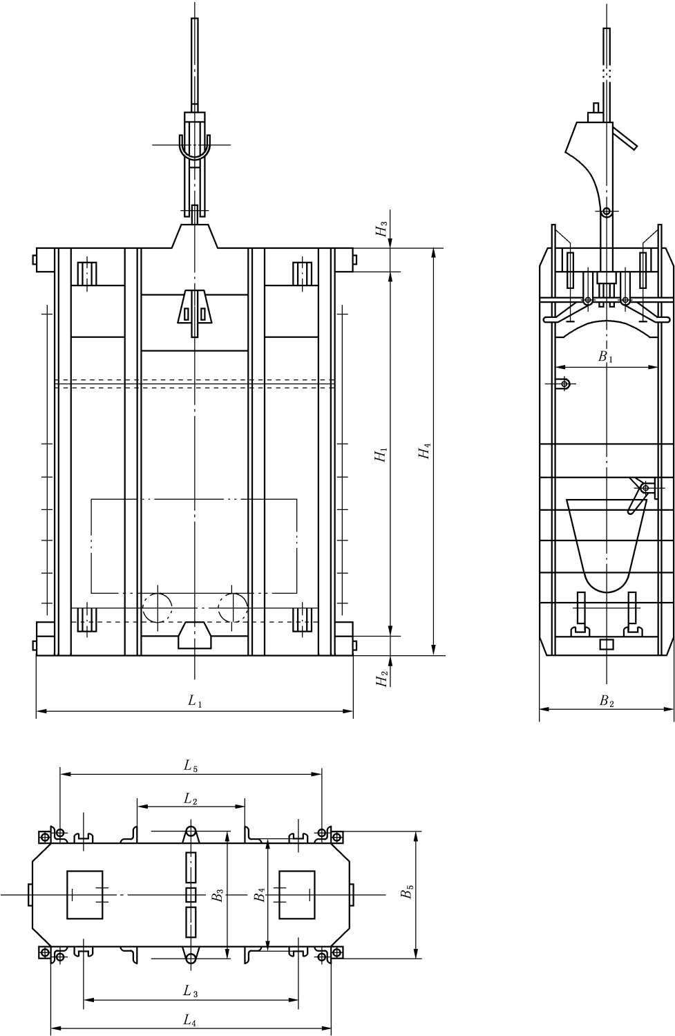
图 2 0.5t 矿车一层一车钢丝绳罐道罐笼
