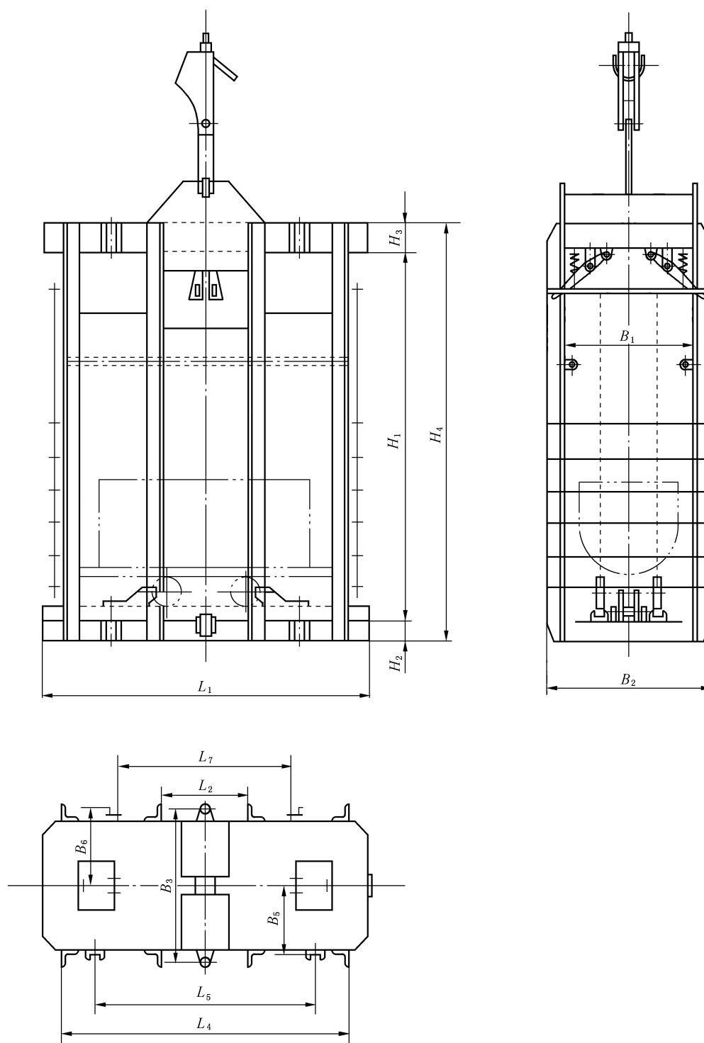
图 3 1t 矿车一层一车钢轨罐道罐笼
