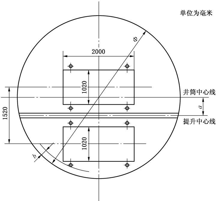
图 C.2 0.5t 矿车一层一车钢丝绳罐道罐笼
