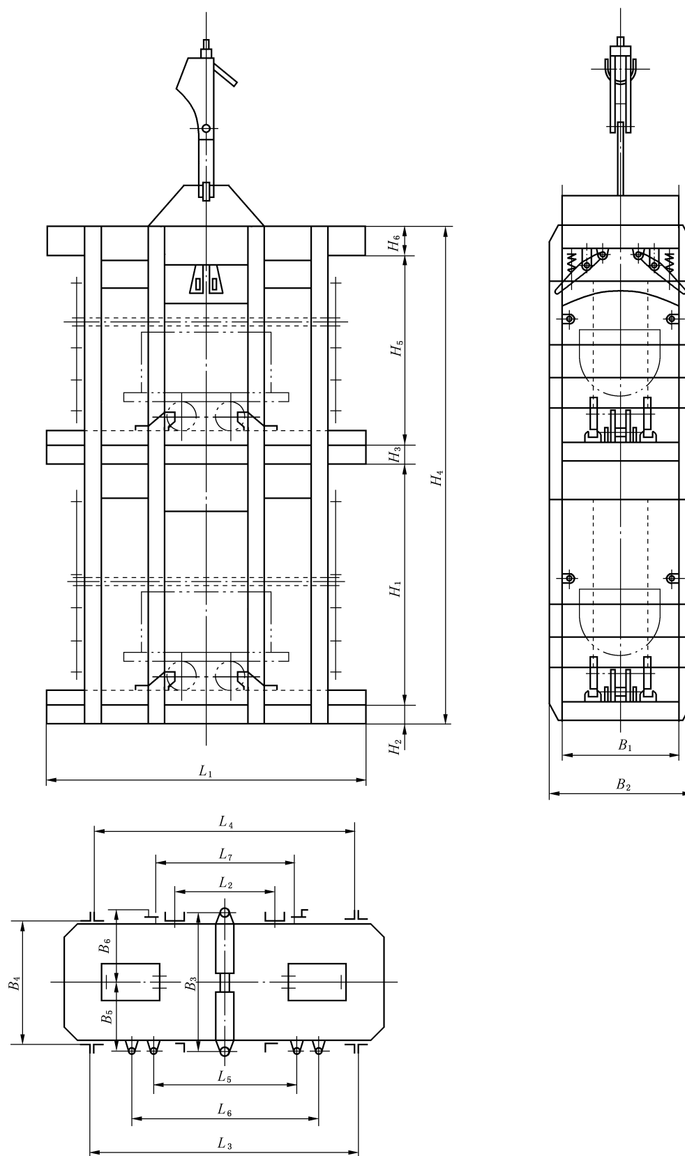
图 7 1t 矿车二层二车钢丝绳罐道罐笼
