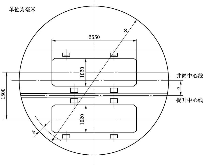
图 C.3 1t 矿车一层一车钢轨罐道罐笼
