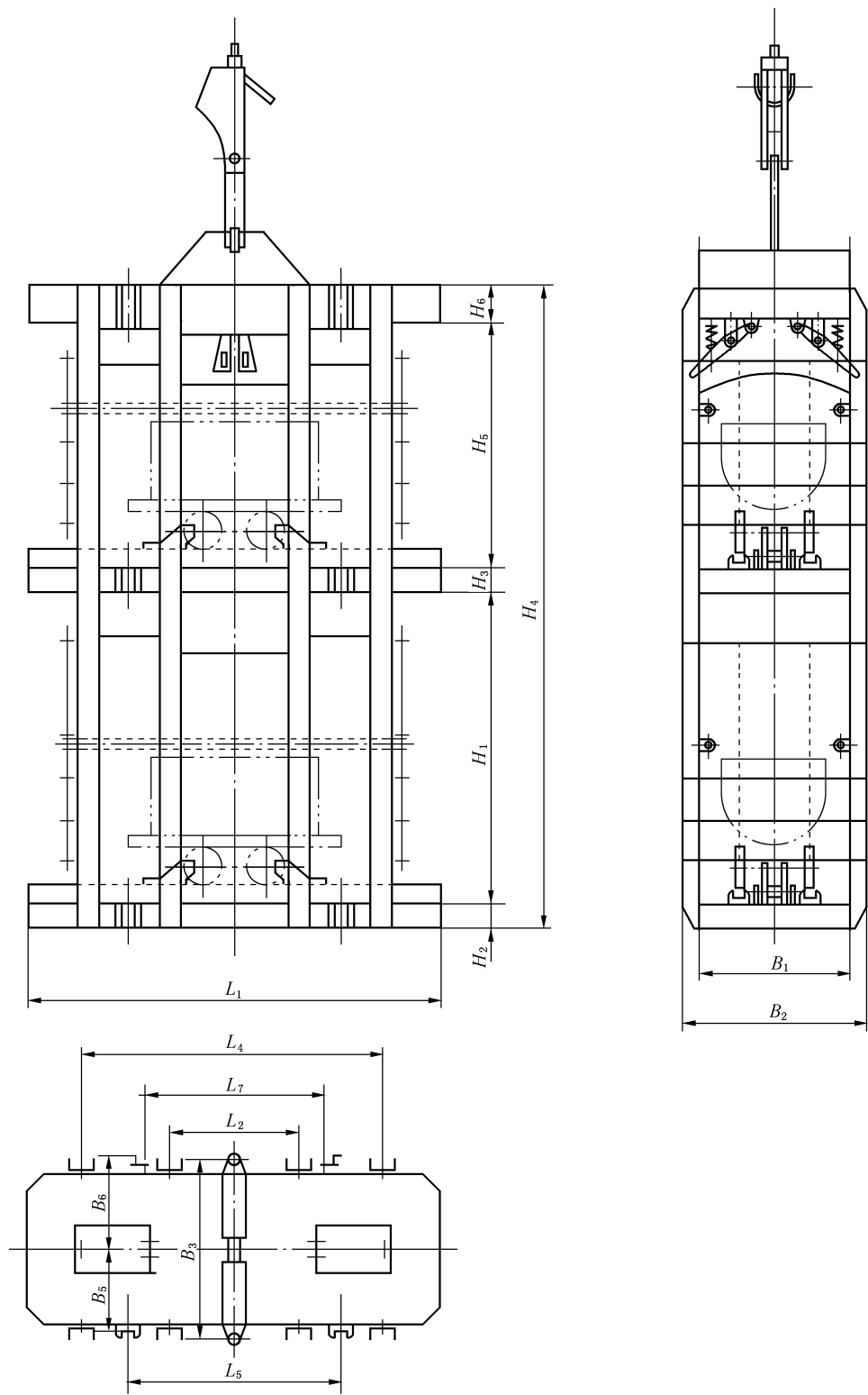
图 6 1t 矿车二层二车钢轨罐道罐笼
