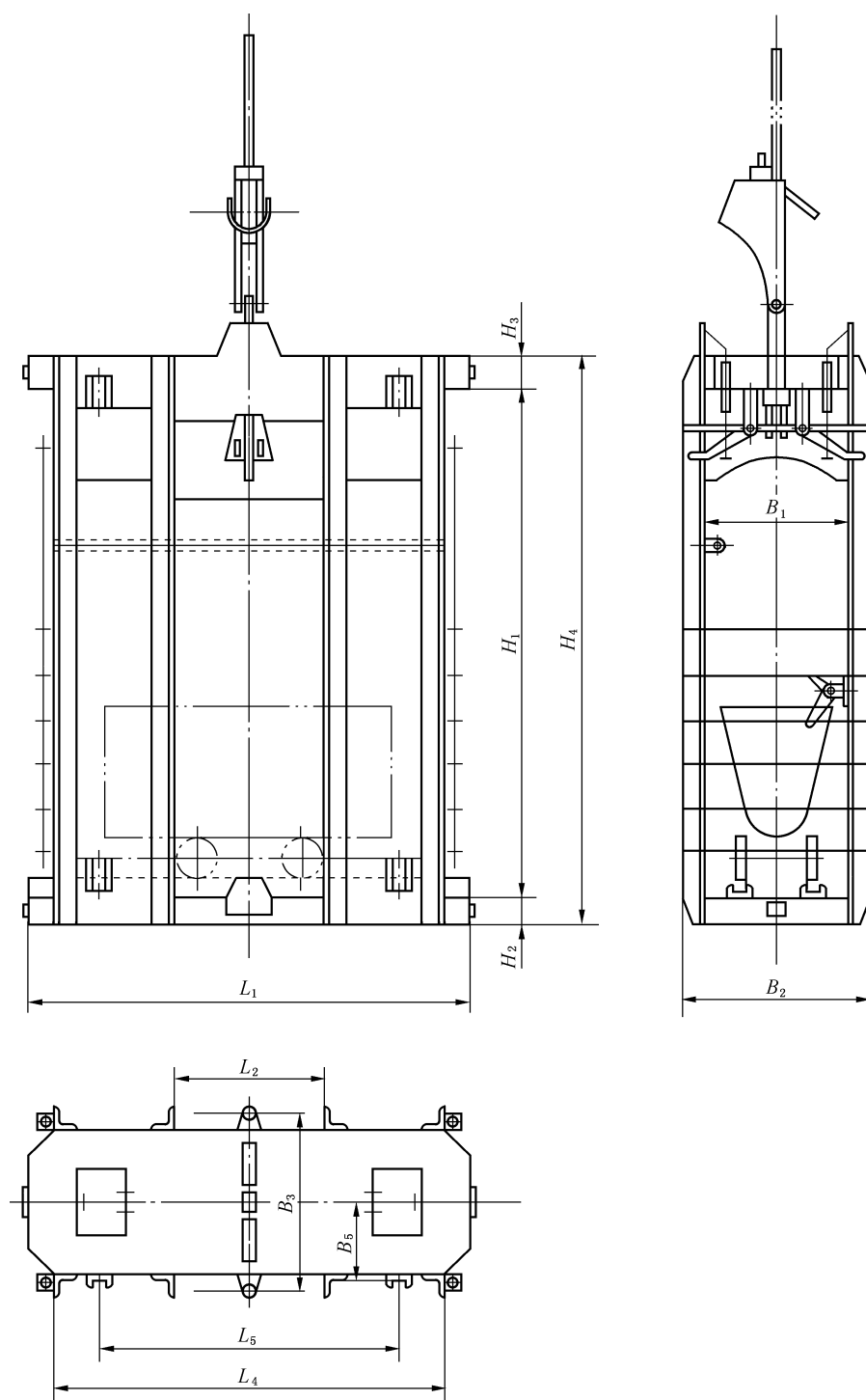
图 1 0.5t 矿车一层一车钢轨罐道罐笼
