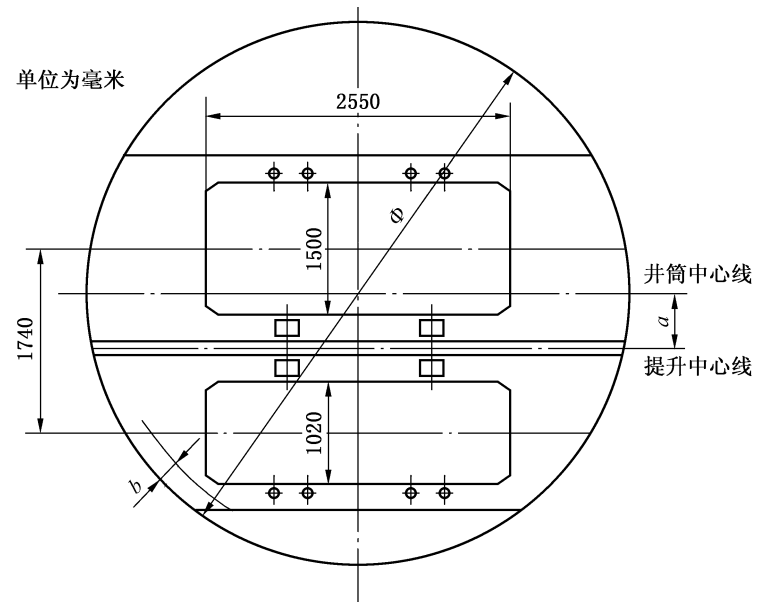
图 C.7 1t 矿车二层二车钢丝绳罐道罐笼
