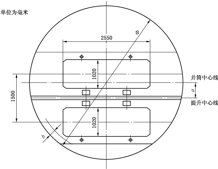
图 C.4 1t 矿车一层一车钢丝绳罐道罐笼
