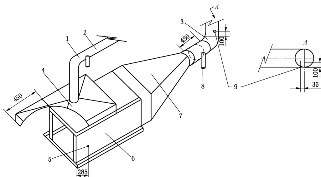
(a) 轴测图
