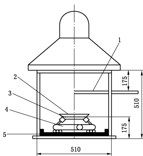
(b)主视图
