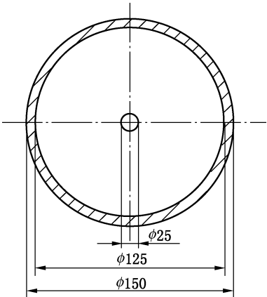
图 D. 1 涂胶区域俯视示意图
