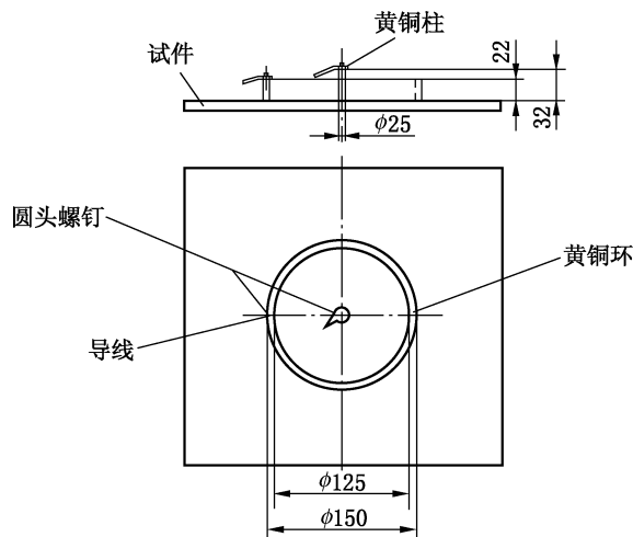
图 D.2 电极尺寸示意图
