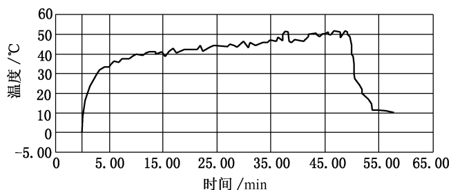
图 G.5 典型排气温度校准曲线
