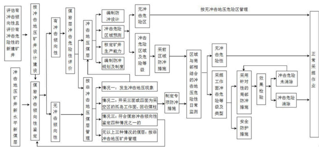
防治煤矿冲击地压基本流程示意图
