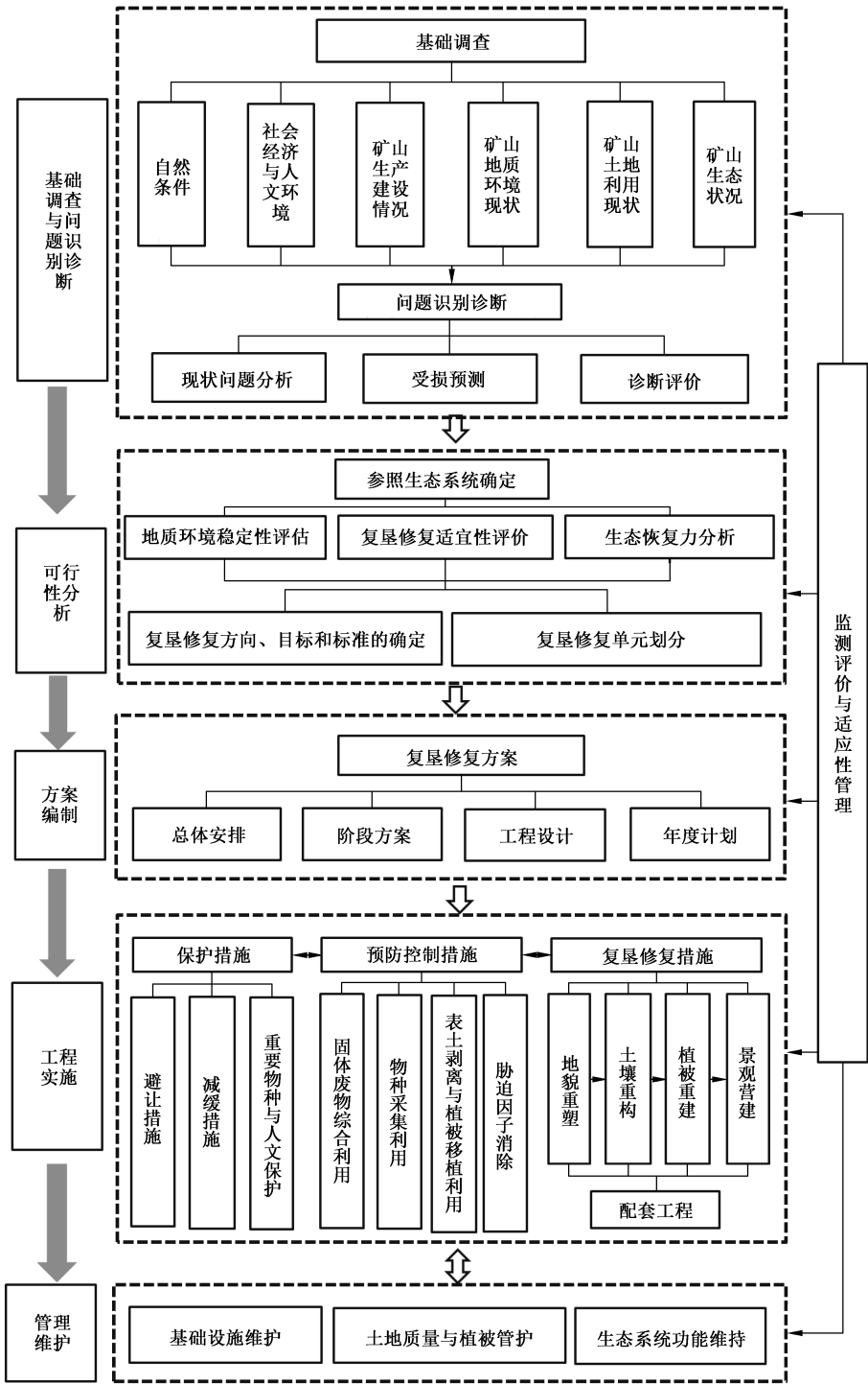
图 1 煤矿土地复垦与生态修复技术路径
