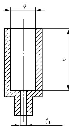
图 2 装药杯示意图
