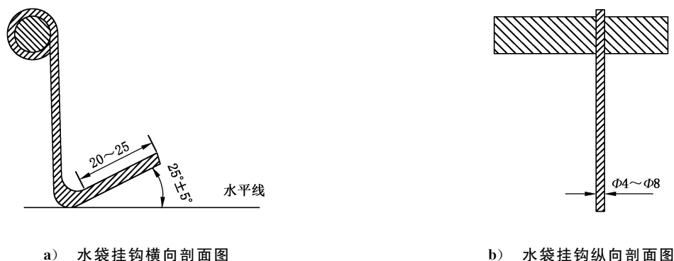
图 3 水袋挂钩图
