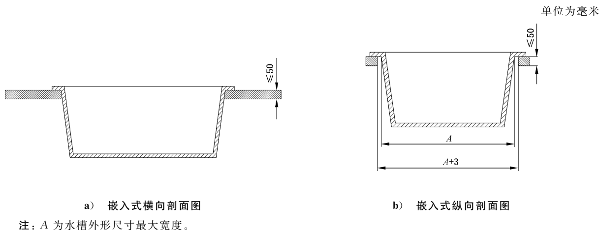
图 1 嵌入式安装
