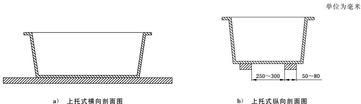
图 2 上托式安装
