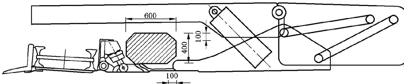
图 1 最小行人通道
