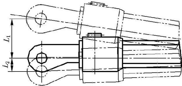
图 3 连接头
