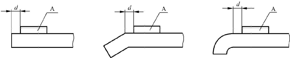
A——垫块; d——垫块与结构件边缘的距离,其值为(20~50)mm。
