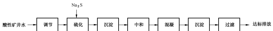
图 D.12 含其他重金属酸性矿井水硫化-中和法基本处理工艺
