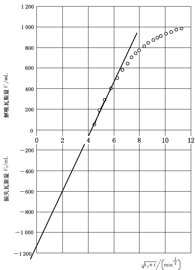
图3 瓦斯损失量计算图
