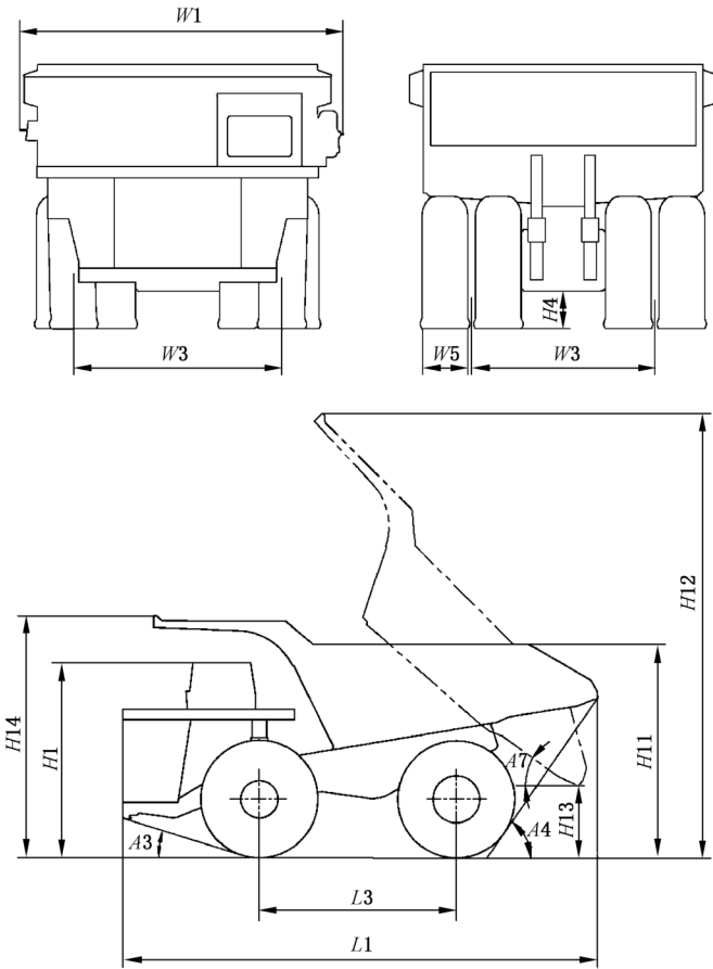
图 1 外形示意图
