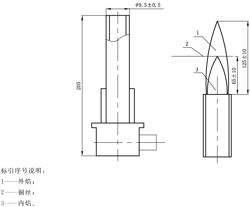
图 G.3 喷灯结构和喷灯火焰
