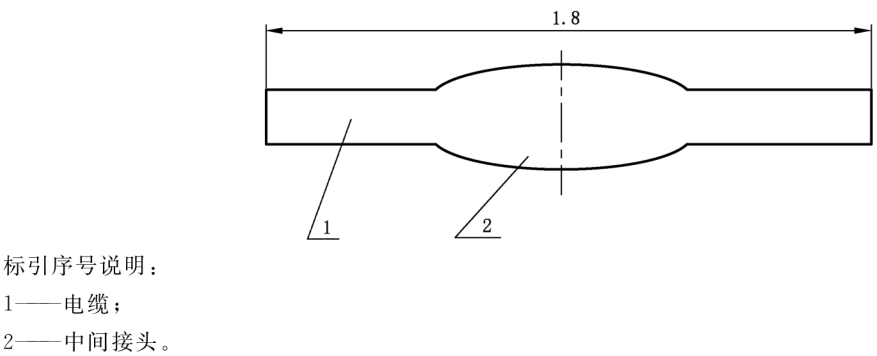
图 G.4 中间接头试样
