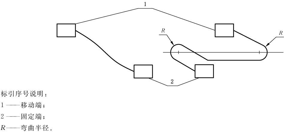
图 E.1 试验机原理
