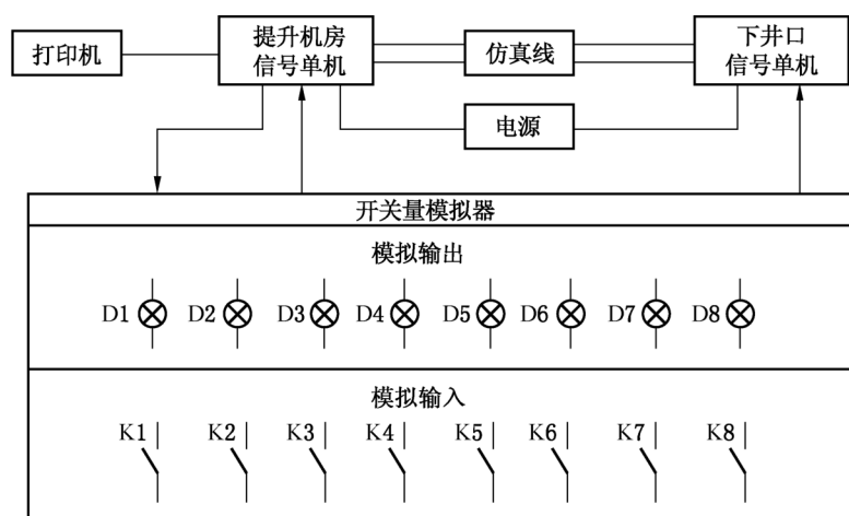
图 1 主井提升信号装置基本性能试验线路
