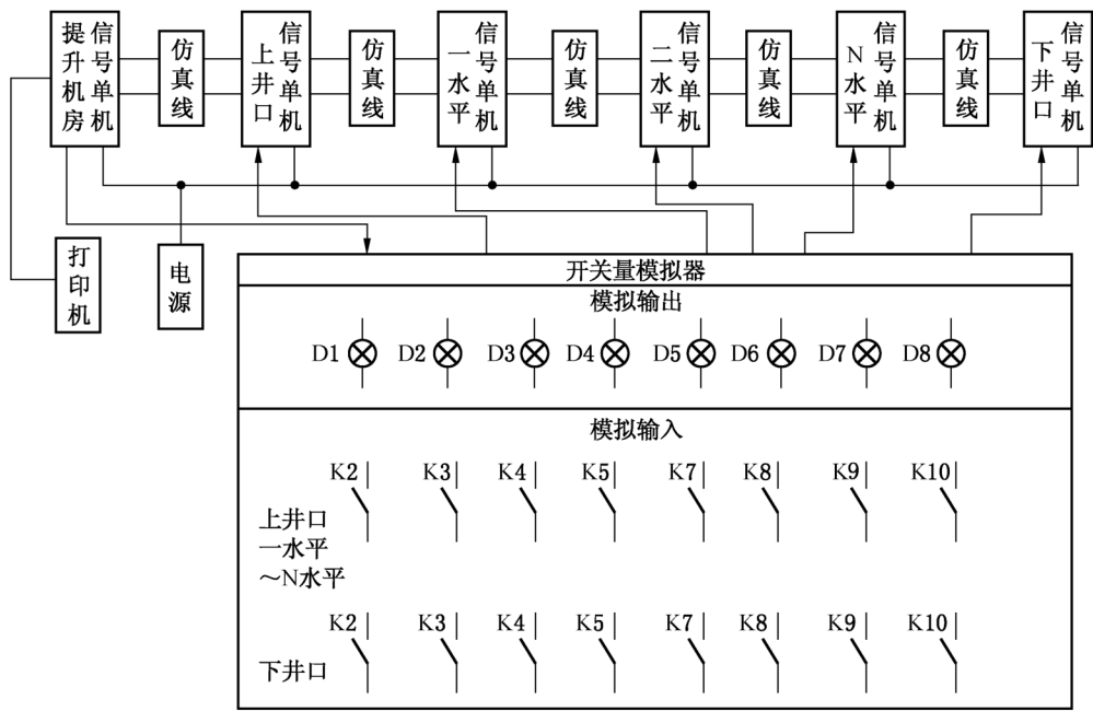
图 2 副井提升信号装置基本试验线路
