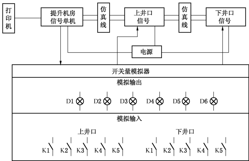
图3 斜井提升信号装置
