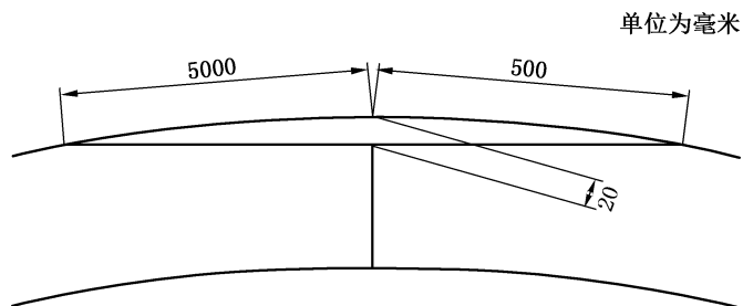
图 1 输送带接缝
