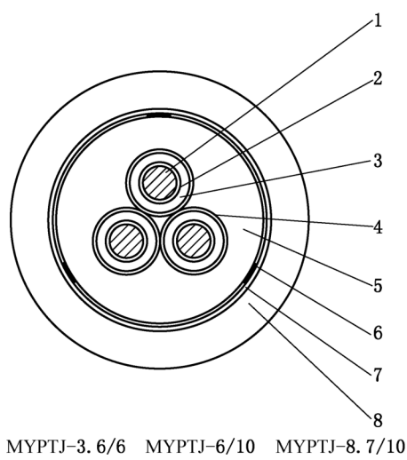
1—动力线芯导体；2—导体屏蔽；3—绝缘；4—绝缘屏蔽(兼做接地线)； 5—内护套；6—监视线芯及半导电带包层；7—绝缘包带；8—外护套
