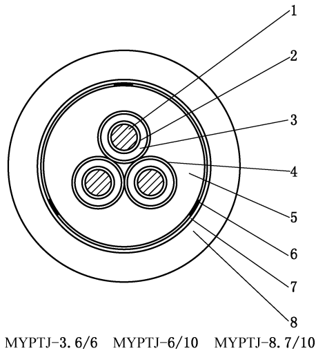
1—动力线芯导体；2—导体屏蔽；3—绝缘；4—绝缘屏蔽（兼做接地线）； 5—内护套；6—监视线芯及半导体包层；7—绝缘包带；8—外护套
