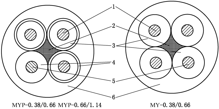
1—动力线芯导体；2—填充；3—绝缘；4—半导电层；5—地线芯导体；6—护套
