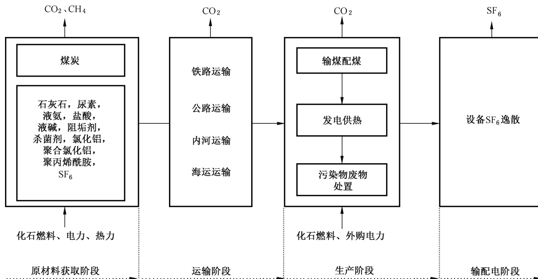
图 1 燃煤发电产品系统边界示意图
