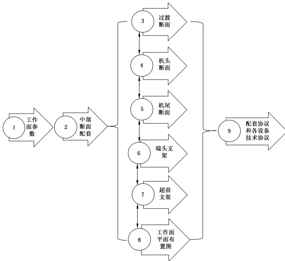
图 2 配套流程图
