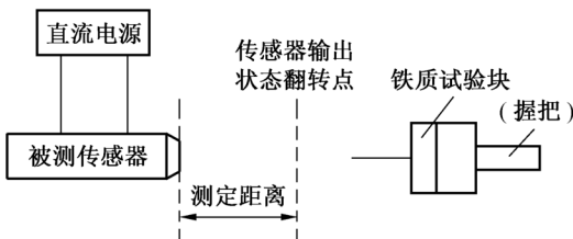
图 2 动作误差试验接线示意图
