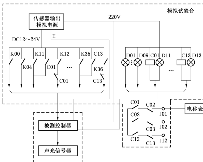
图 1 基本功能试验接线示意图
