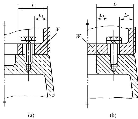
图 3 平面式
