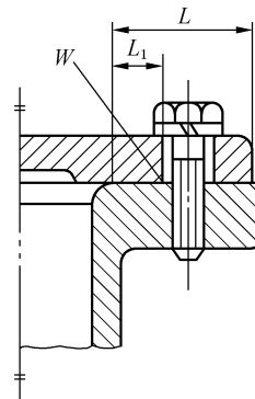
图 2 平面式
