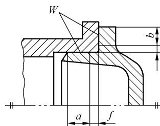
图 5 止口式
