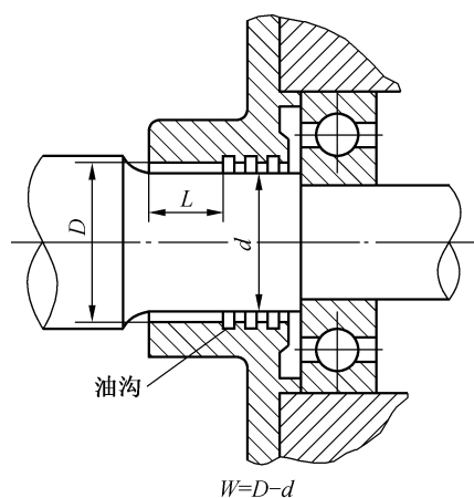
图 6 圆筒式
