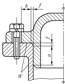
图 4 止口式
