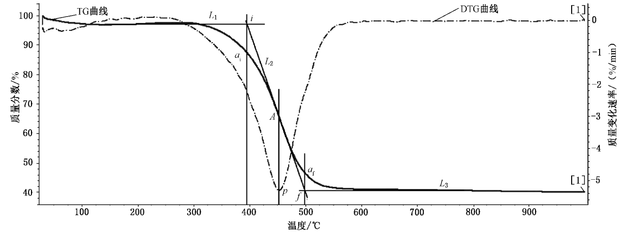
图 2 煤炭燃烧 TG-DTG 曲线
