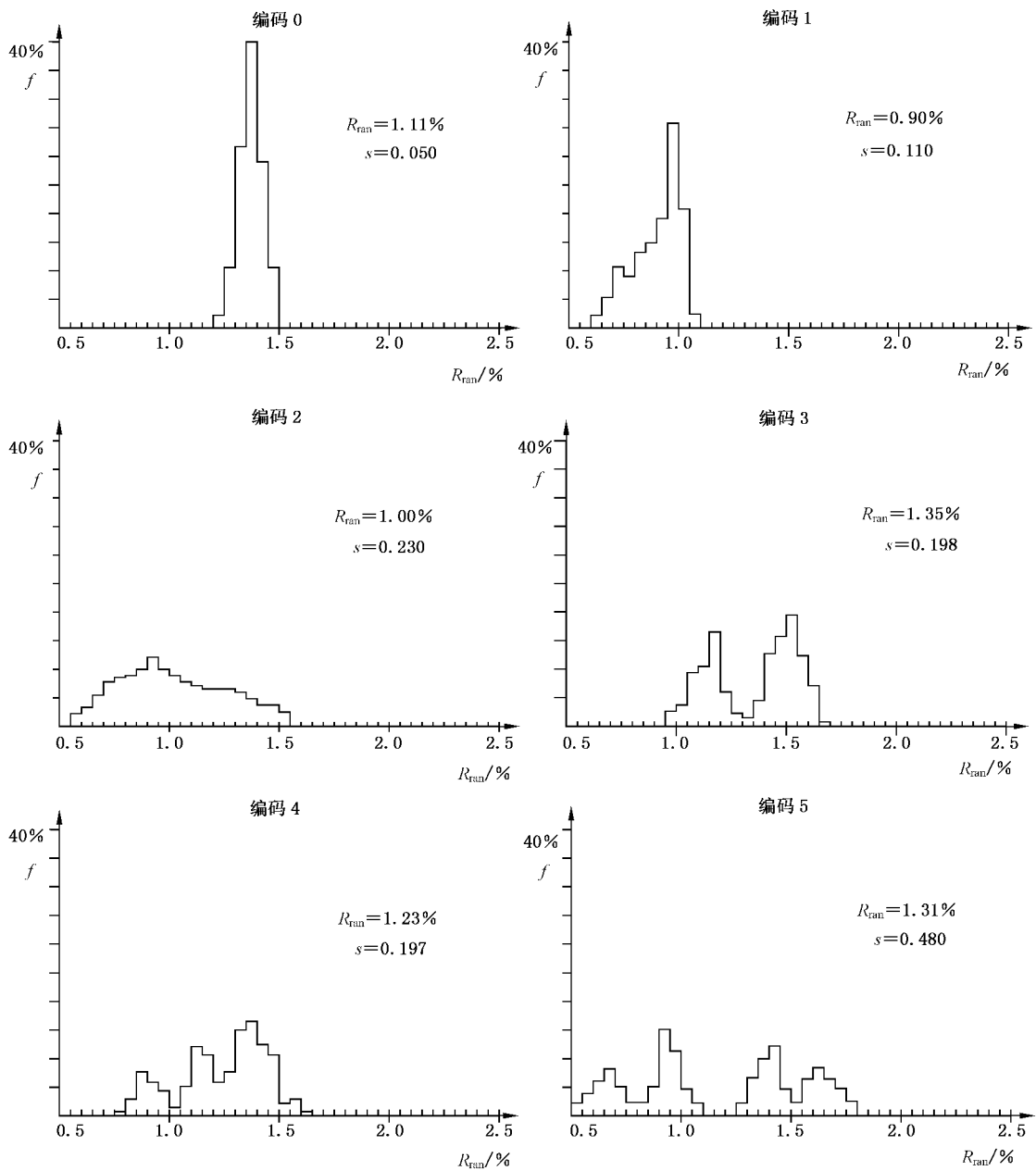
图 A.1 各种混煤类型的商品煤镜质体反射率频率分布图示例
