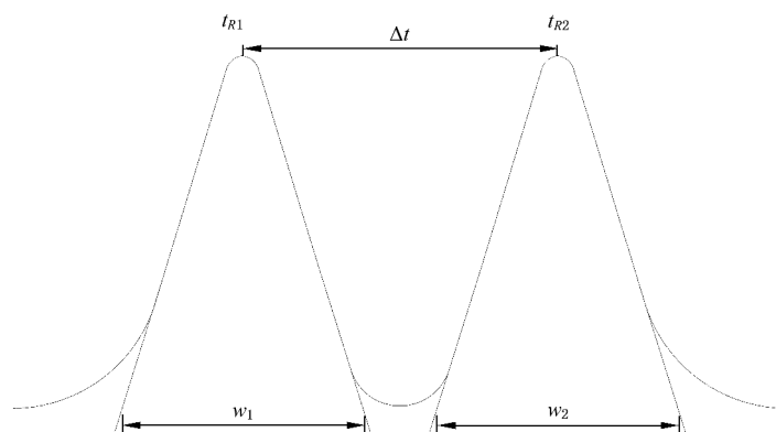
图 2 色谱柱的分离度
