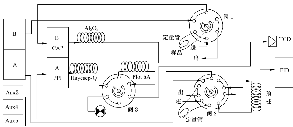
图 1 气相色谱仪系统连接图
