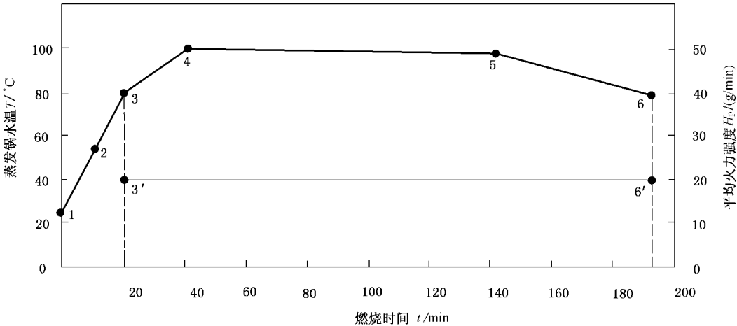
图 1 燃烧特性曲线图
