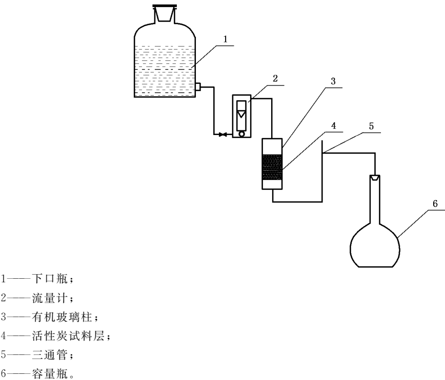
图 A.1 腐殖酸吸附试验装置图
