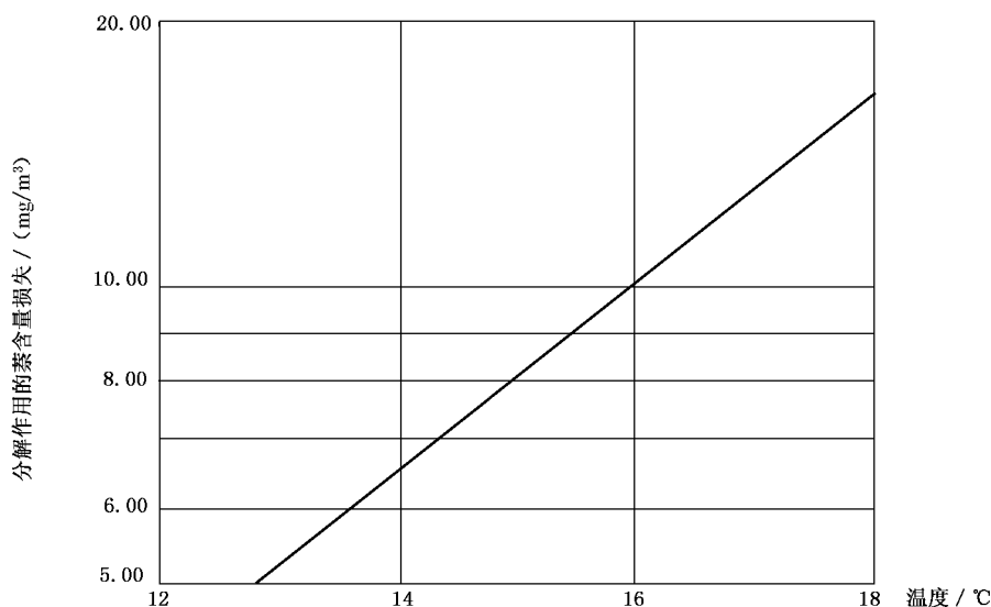
图 6 13 °C ~ 18 °C 下实测萘含量损失校正值图
