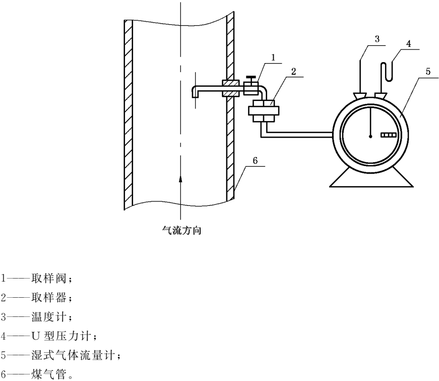
图 3 测定焦油和灰尘含量的取样装置图
