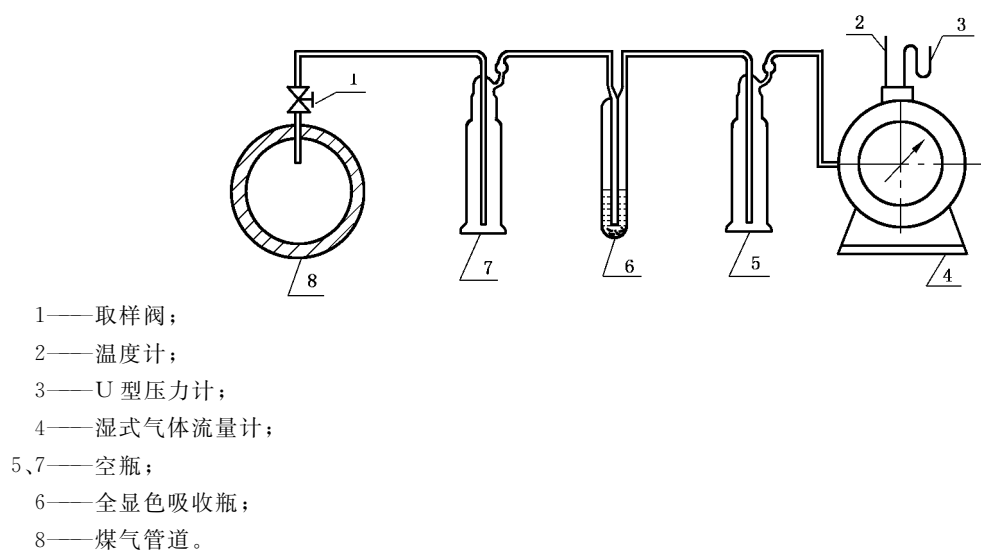
图 15 分光光度法测定 \text{H}_2\text{S} 含量取样装置图
