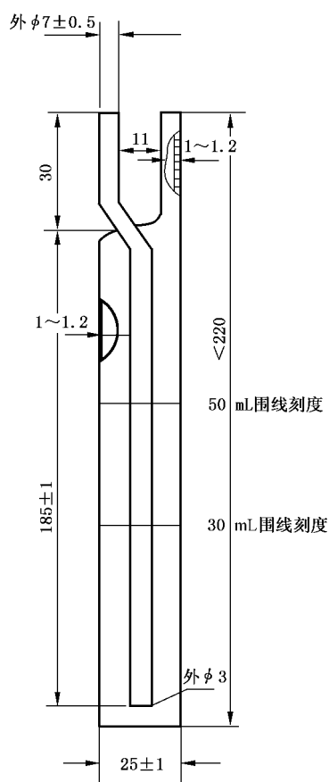
图 14 全显色吸收瓶规格图
