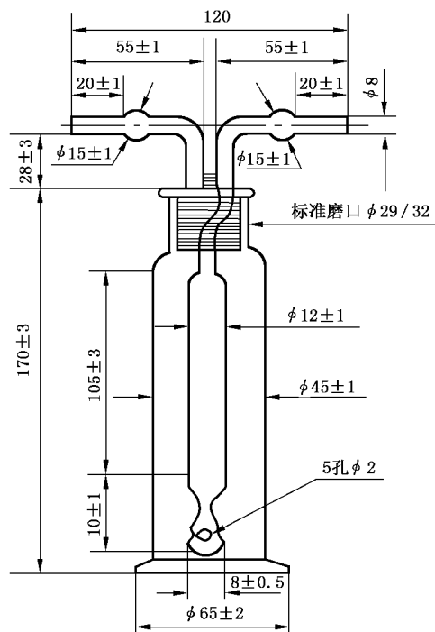
图 10 洗气瓶规格图
