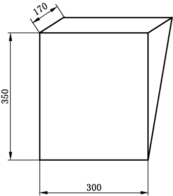
图 A.4 风斗示意图
