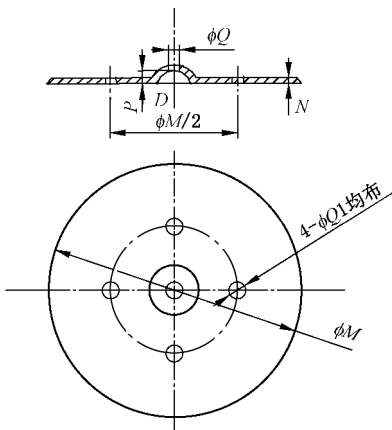
图 5 封火盖示意图
