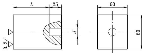
图2 平面参考试块示意图
